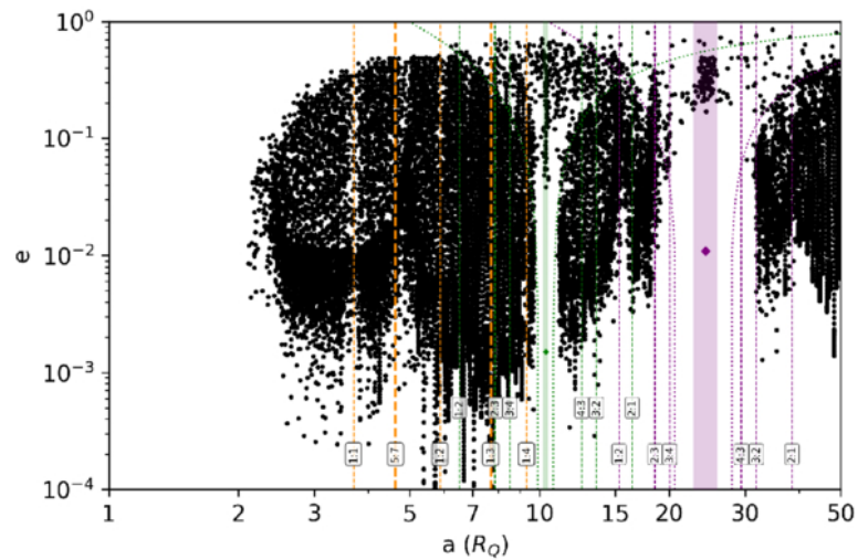
(d) 10^4 T_Q
