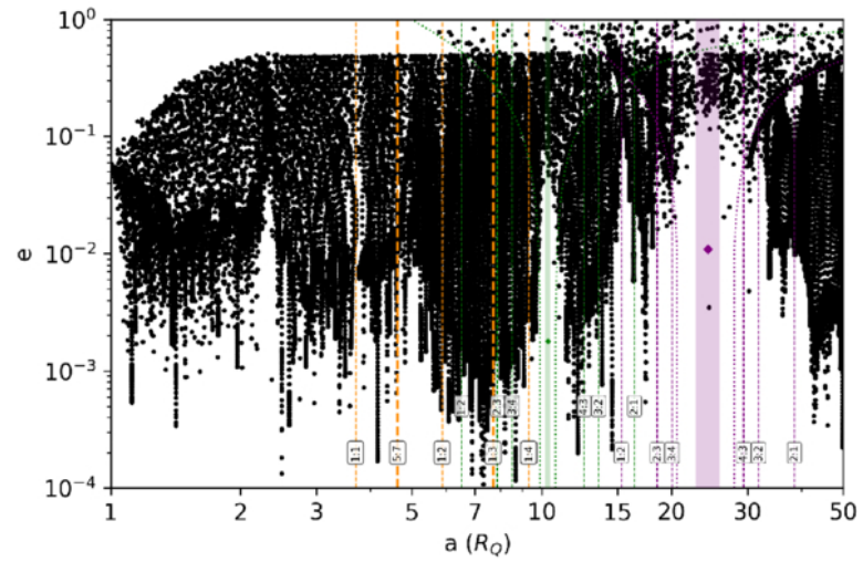
(b) 10^2 T_Q
