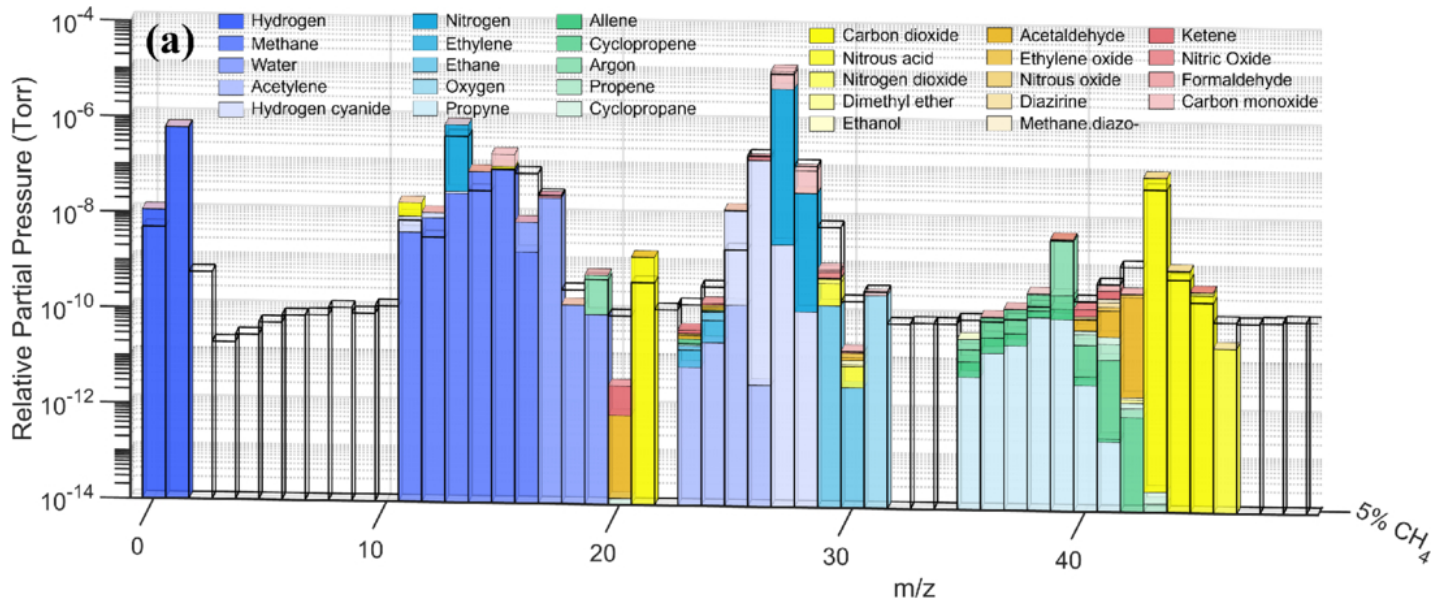
Figure 1. from Zhengbo Yang et al 2026 Planet. Sci. J. 7 doi:10.3847/PSJ/ae5e70 https://dx.doi.org/10.3847/PSJ/ae5e70
