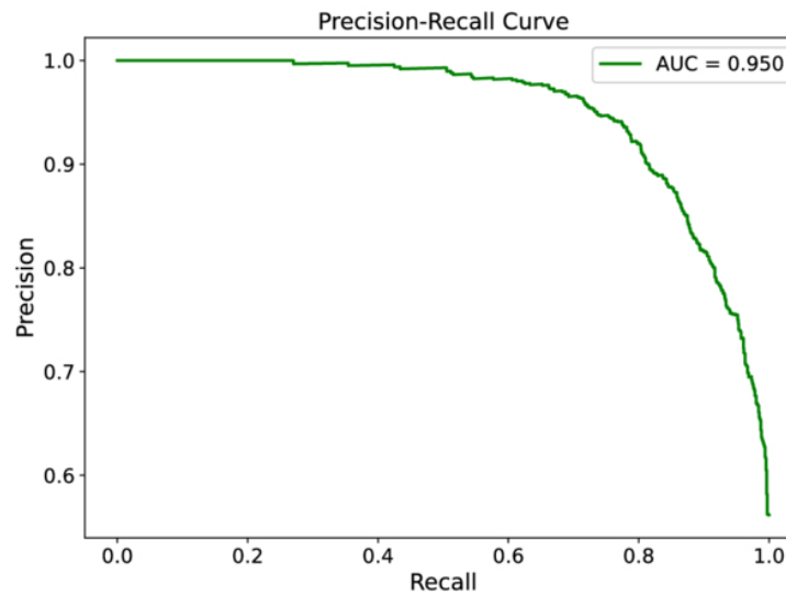
(d) Precision-Recall (PR) curve.
