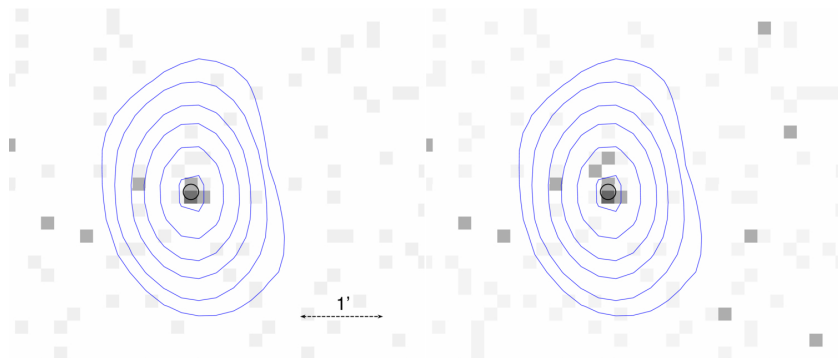
(d) MRC B1827–360 / G4Jy 1487
