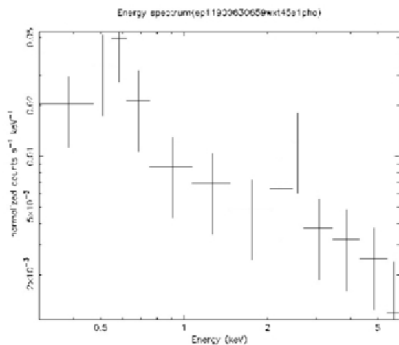
(d) Case 1: PI spectrum
