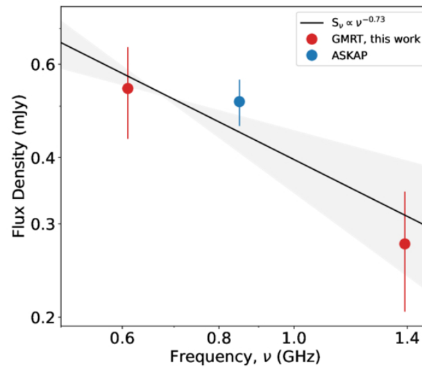
(d) HD 175362
