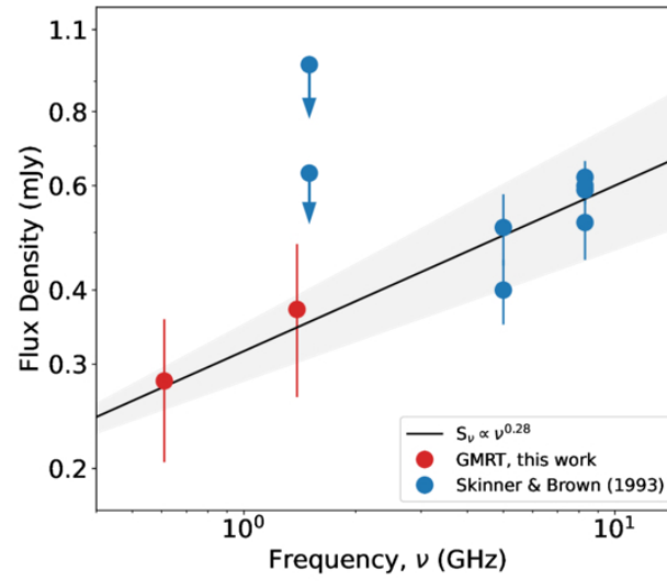
(b) HD 200775
