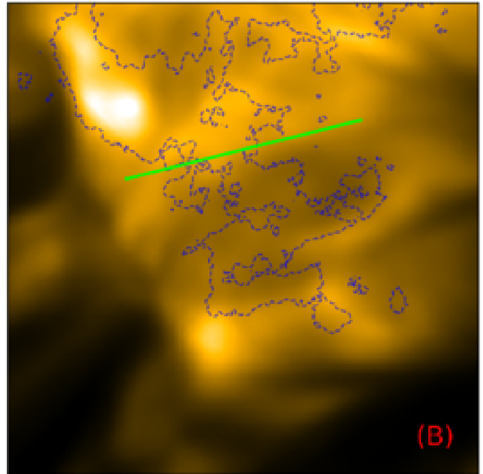
AIA 171 Å [DN/s]
