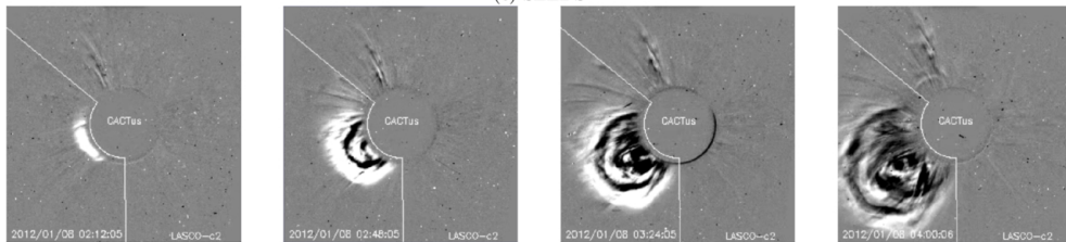
(d) CACTus
