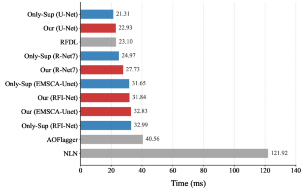
(b) LOFAR
