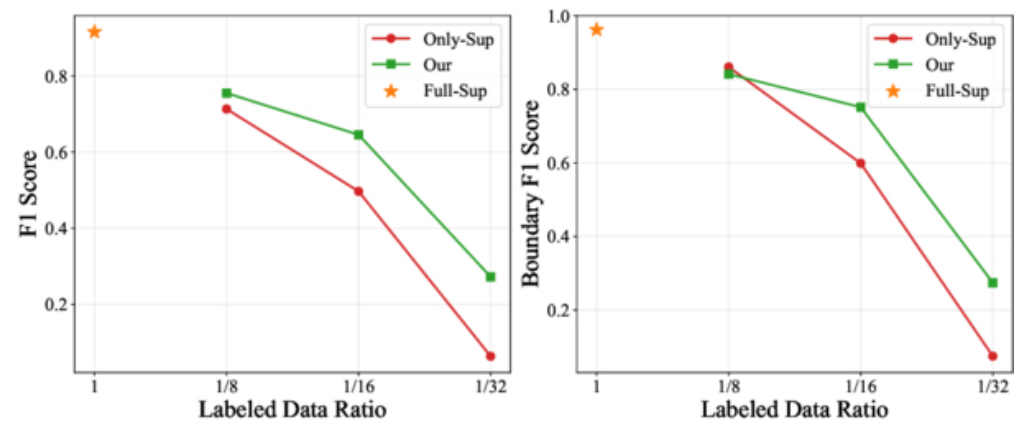
(d) U-Net
