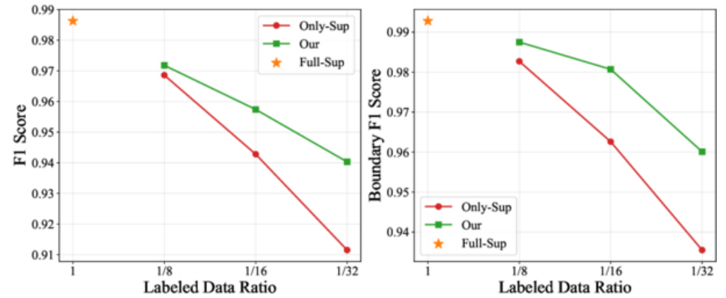
(b) RFI-Net
