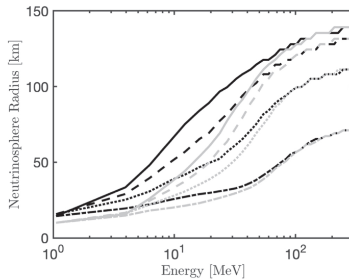
(d) Neutrinosphere Radius
