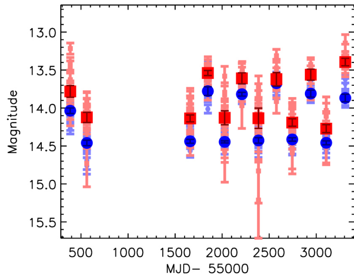
SDSSJ0033+1900
