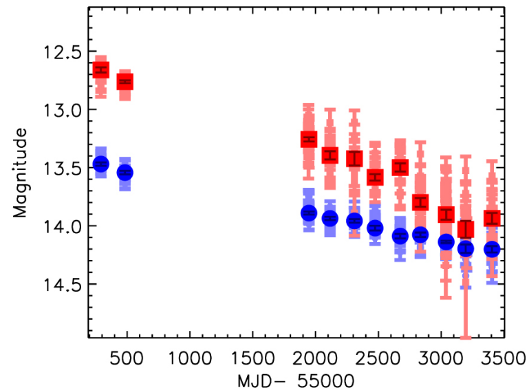
SDSSJ0748+4712
