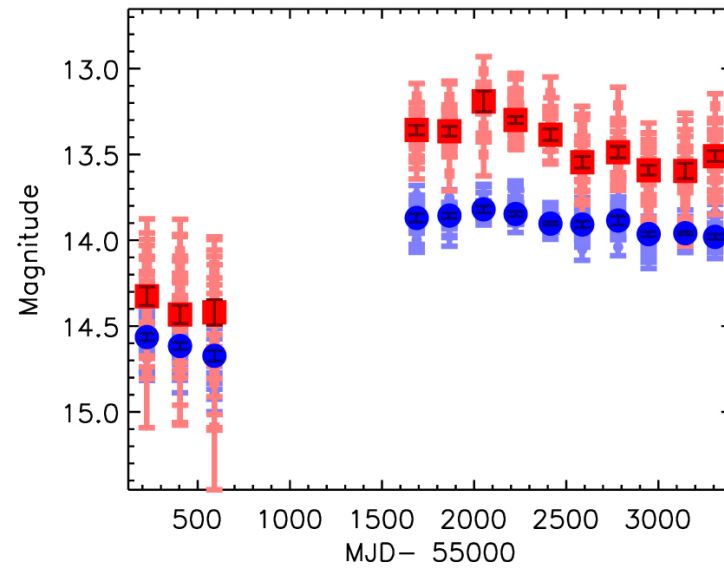
SDSSJ1513+2213
