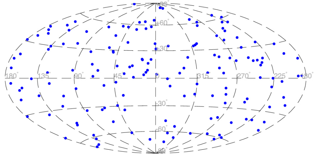
(d) 20-pc census - Y Dwarfs Only
