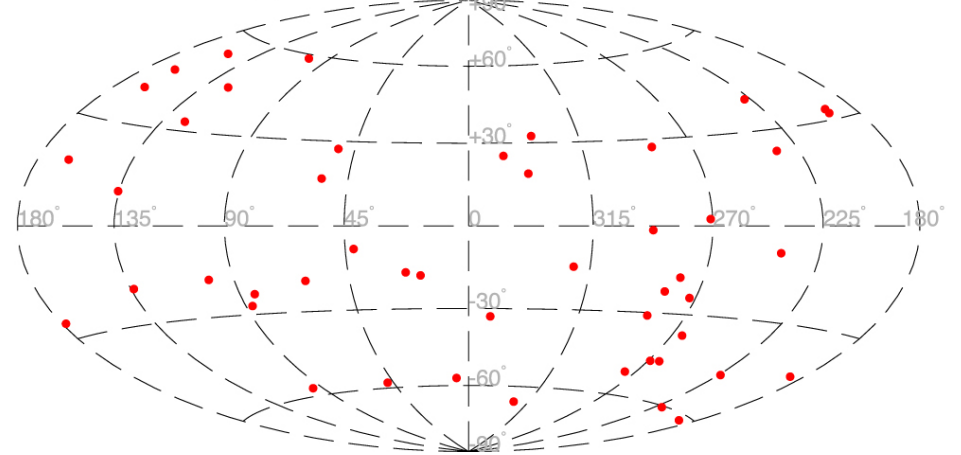
(d) 20-pc census - Y Dwarfs Only
