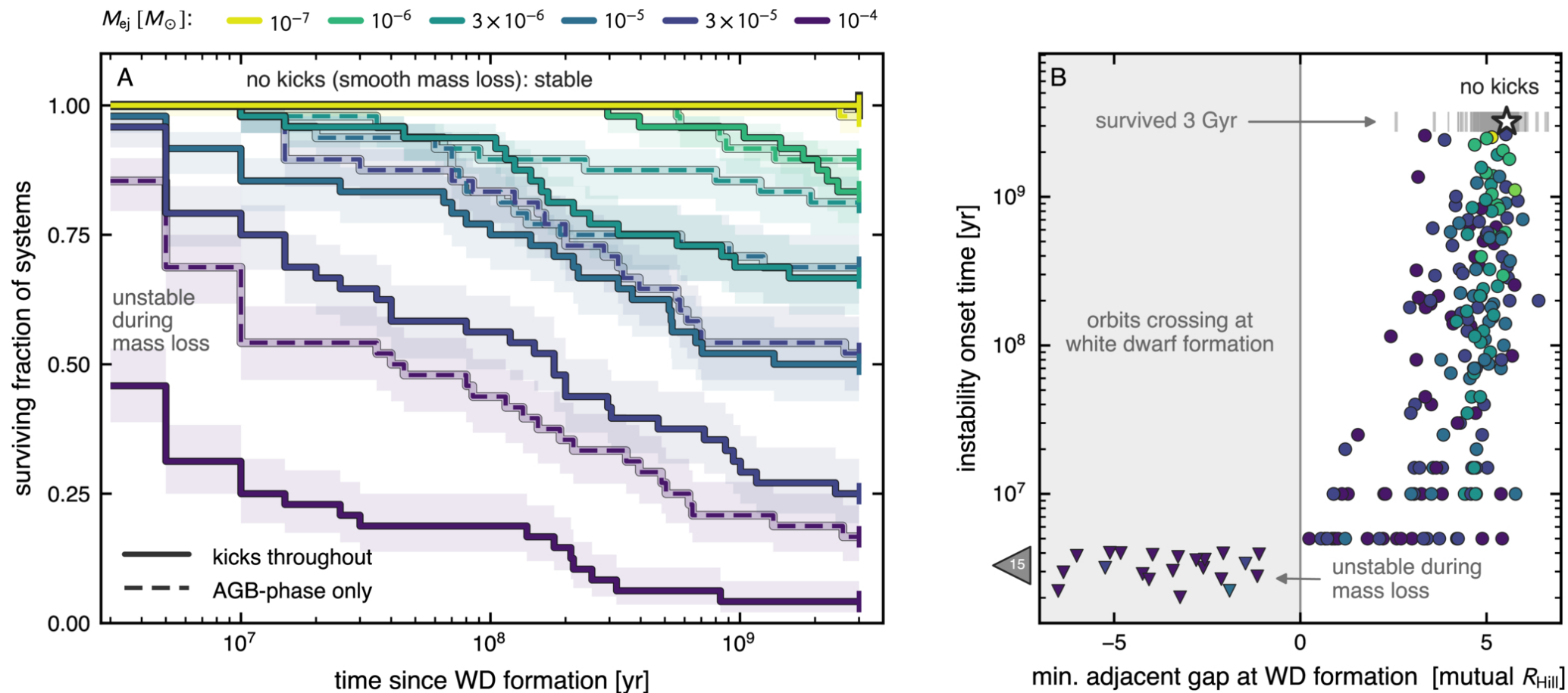
Figure 4. from Konstantin Batygin et al 2026 Astrophys. J. Lett. 1009 doi:10.3847/2041-8213/aea290 https://dx.doi.org/10.3847/2041-8213/aea290
