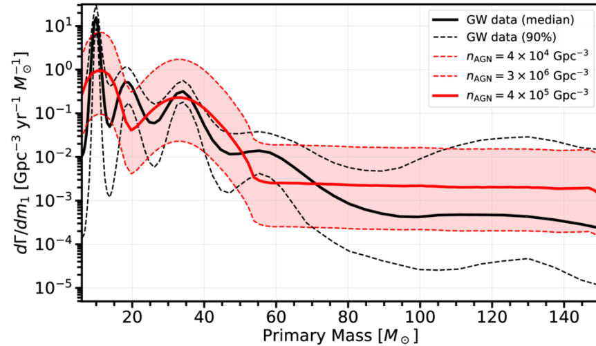
(d) Merger rate ( f_{\text{quiet}} = 70\% )
