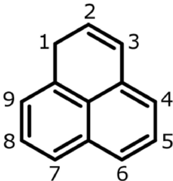
1H-phenalene
