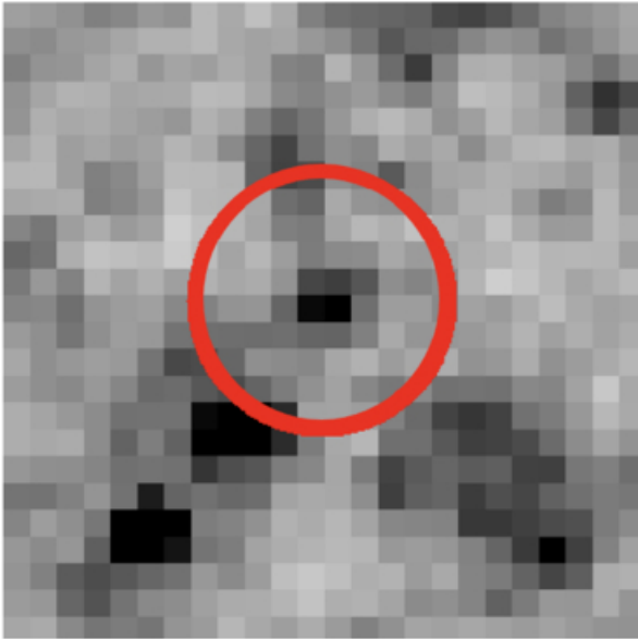
HST WFC3-IR F160W
