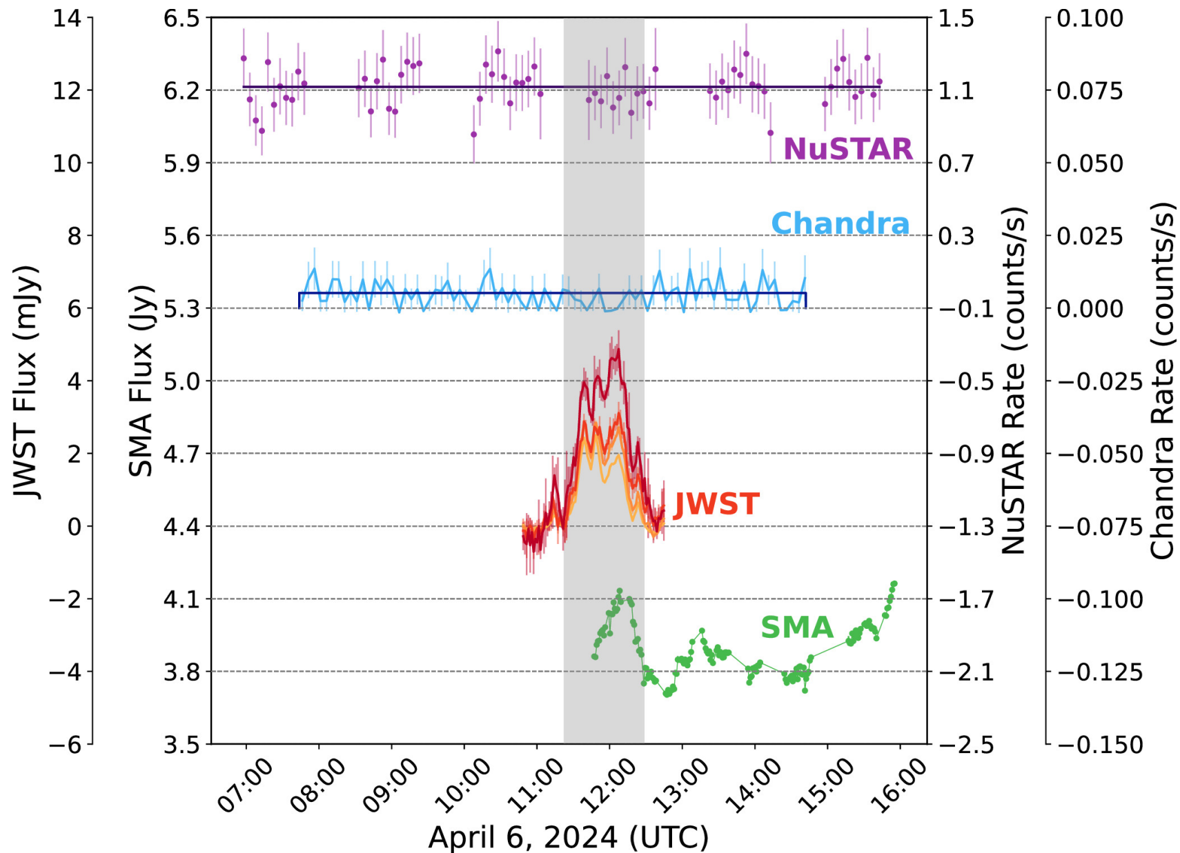
Figure 2. from Sebastiano D. von Fellenberg et al 2025 Astrophys. J. Lett. 979 doi:10.3847/2041-8213/ada3d2 https://dx.doi.org/10.3847/2041-8213/ada3d2
