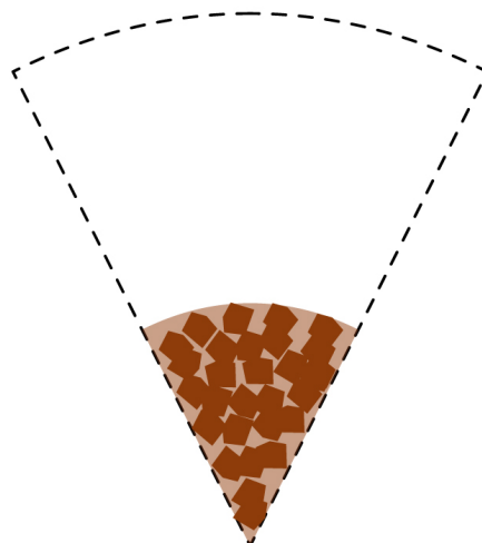
(d) Transformation to asteroid
