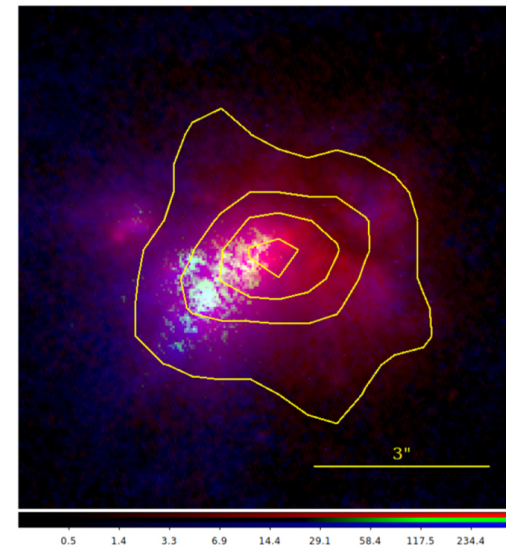
(f) LARS 03
