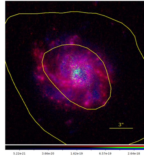
(c) IRAS 08339+6517
