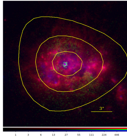
(b) ESO 338-IG004
