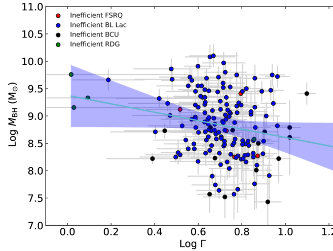
(d) Black hole mass versus bulk Lorentz factor in radiatively inefficient AGNs
