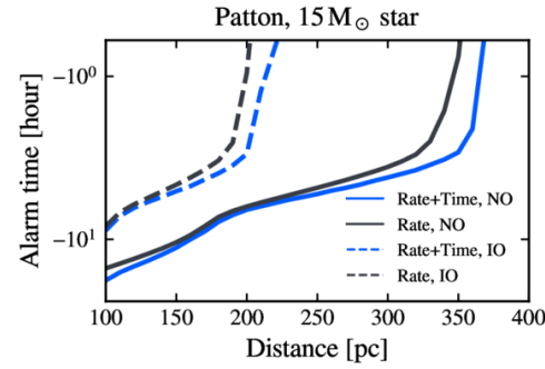
(d) SK, Patton model signal
