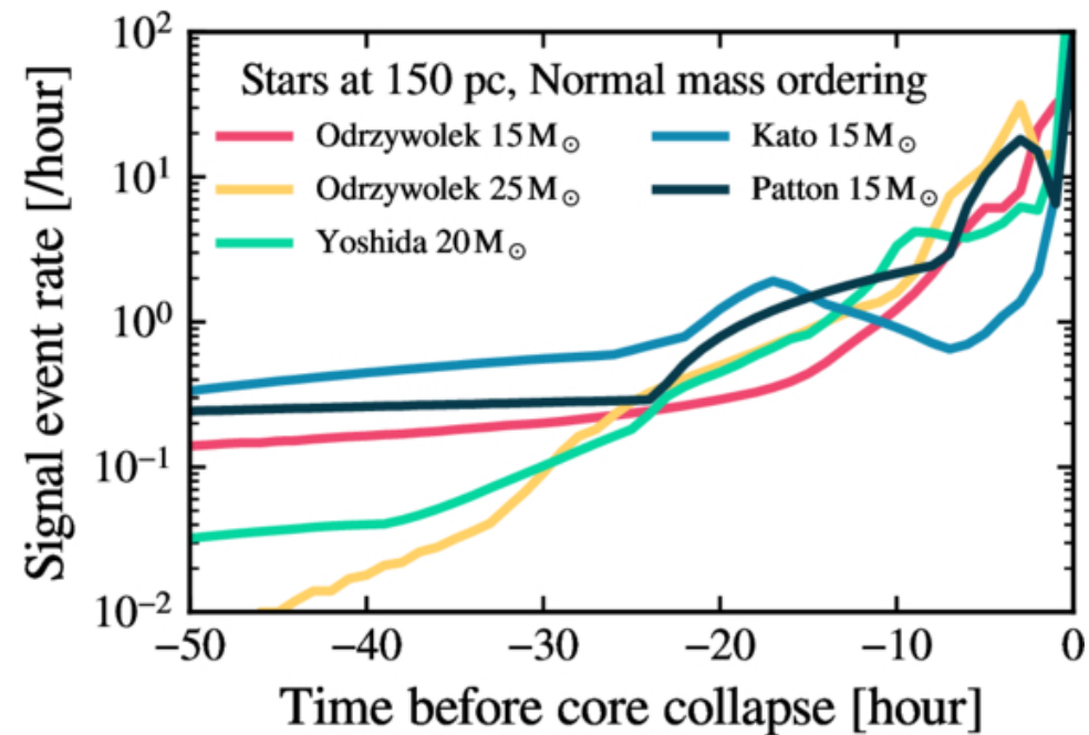
(b) Super-Kamiokande
