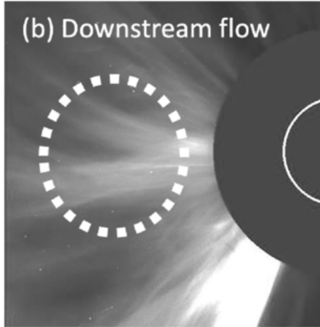
SOHO/LASCO C2 2003/11/18 11:26 UT
