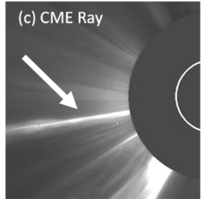
SOHO/LASCO C2 2003/11/18 16:26 UT
