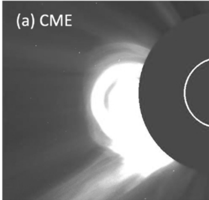
SOHO/LASCO C2 2003/11/18 10:06 UT
