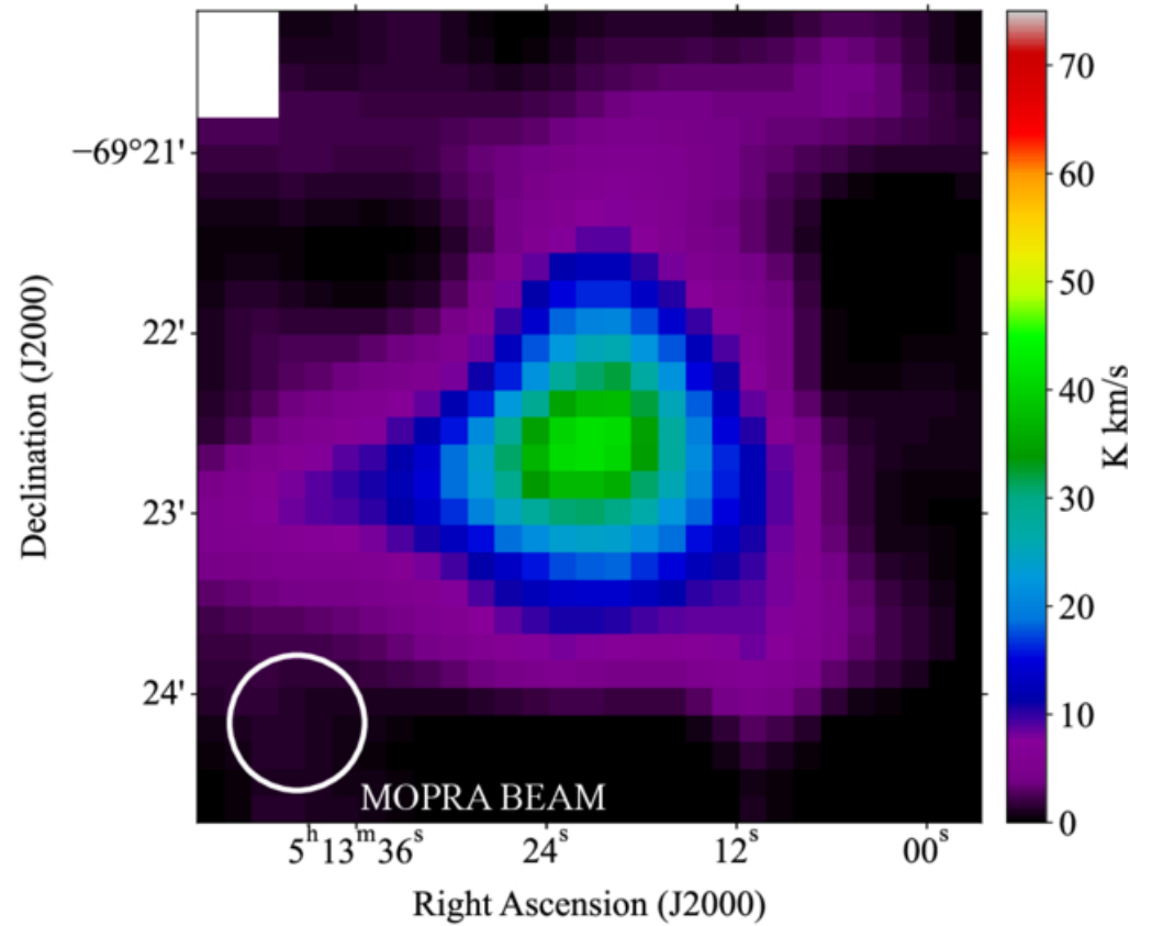
(b) MOPRA CO(J=1-0)
