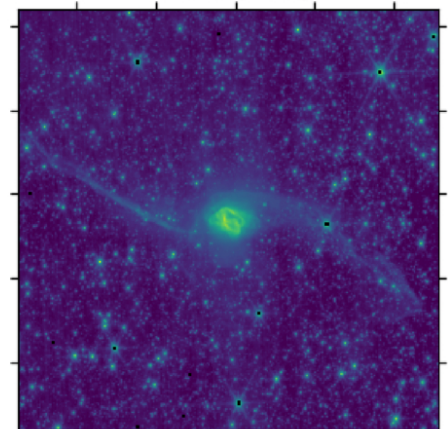
F164N [Fe II]
