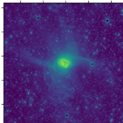
F405N (Br-a)
