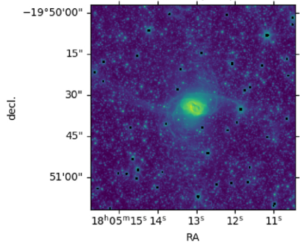
F356W (PAH)
