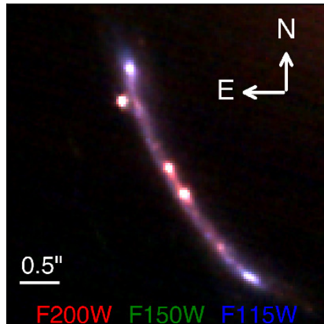
SGAS1723+34
