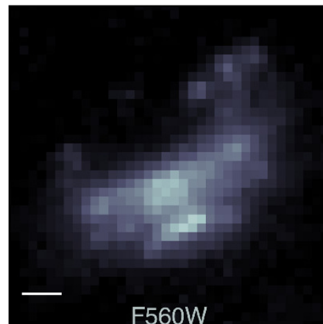
SGAS1226+21
