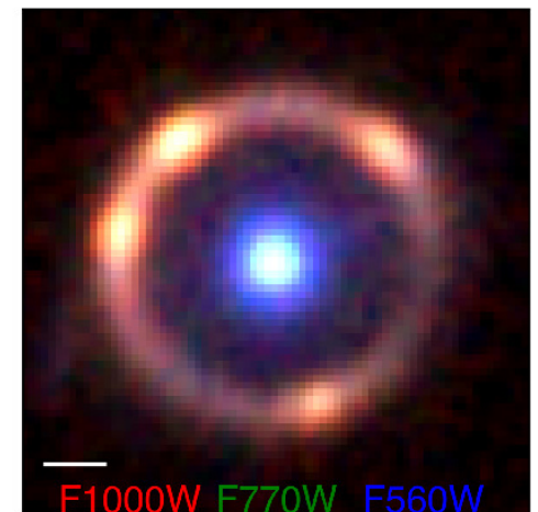
SPT0418-47
