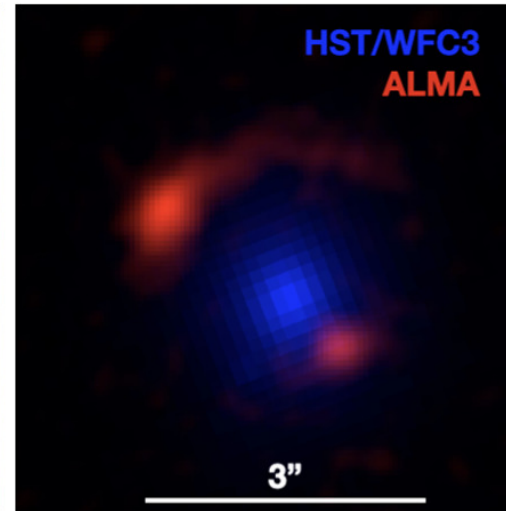
SPT2147-50
