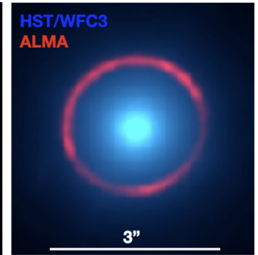
SPT0418-47
