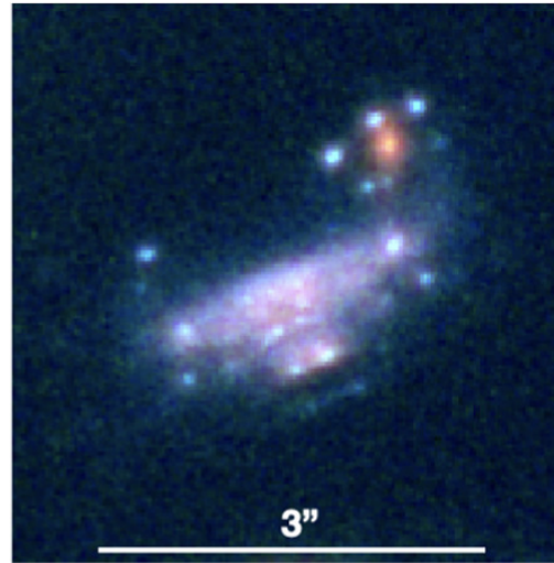
SDSS1226+21
