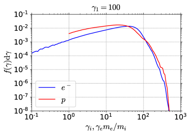
(d) 700 \leq x/(c/\omega_{pe}) \leq 1050
