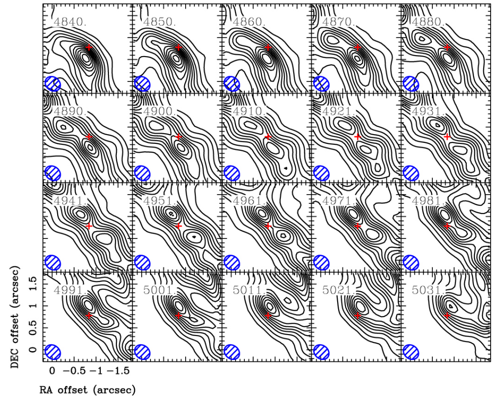
(b) ^{12}\text{CO}(2-1)
