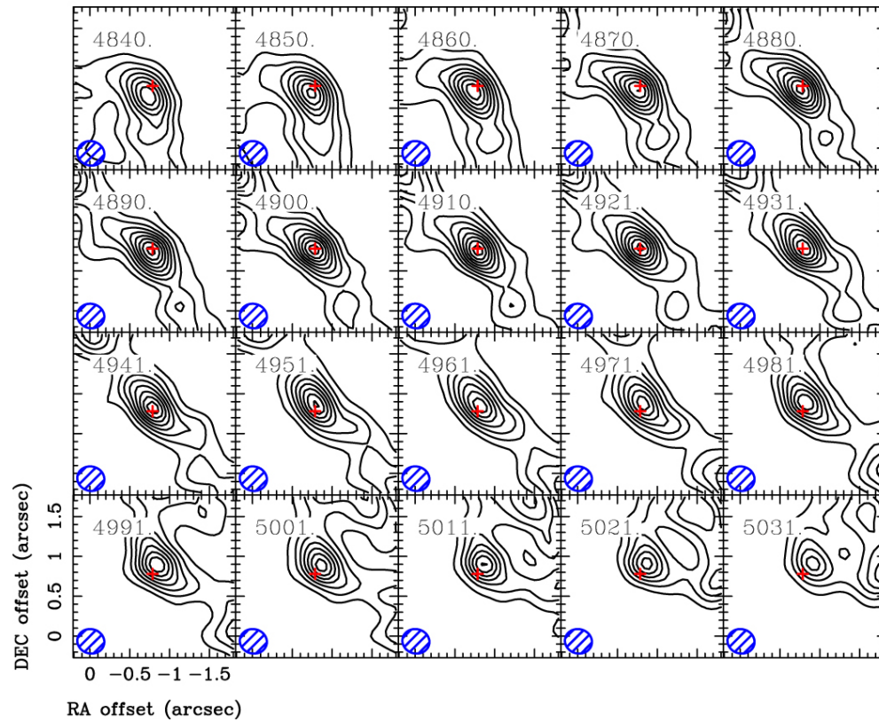
(a) [C I](1-0)
