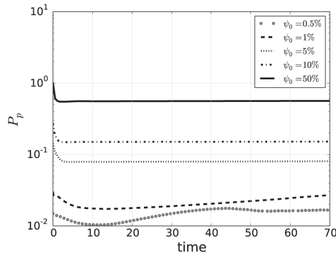
(d) Plasma pressure at the X-point
