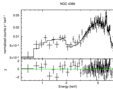
(j) Chandra spectrum.
