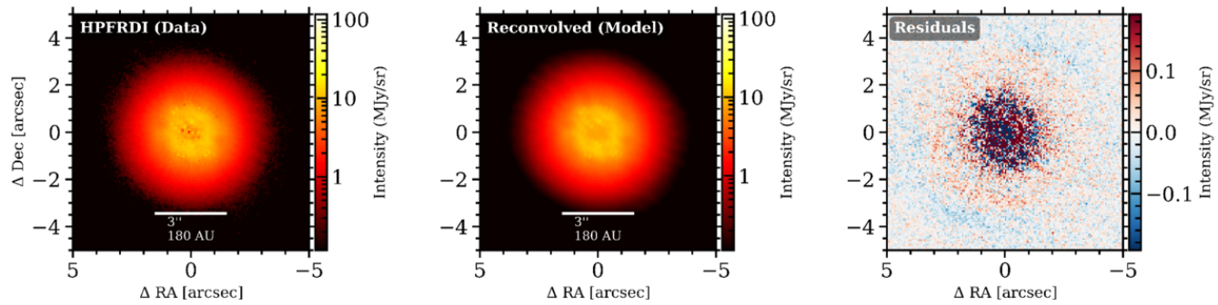
(b) F356W
