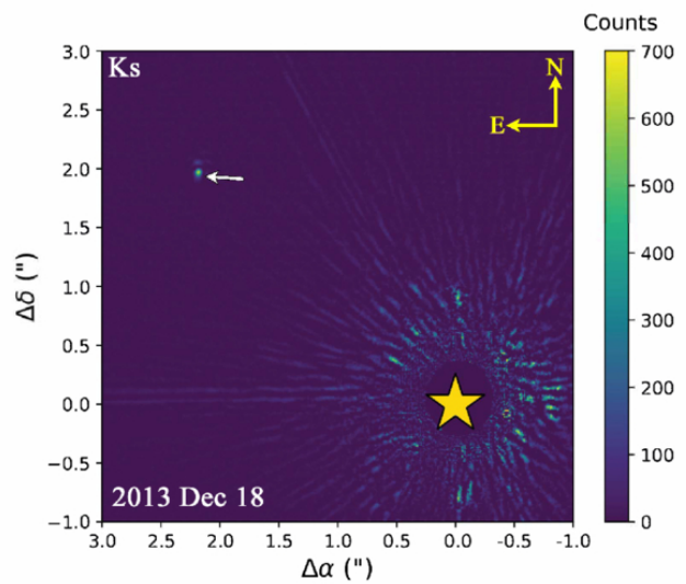
Epoch 1
