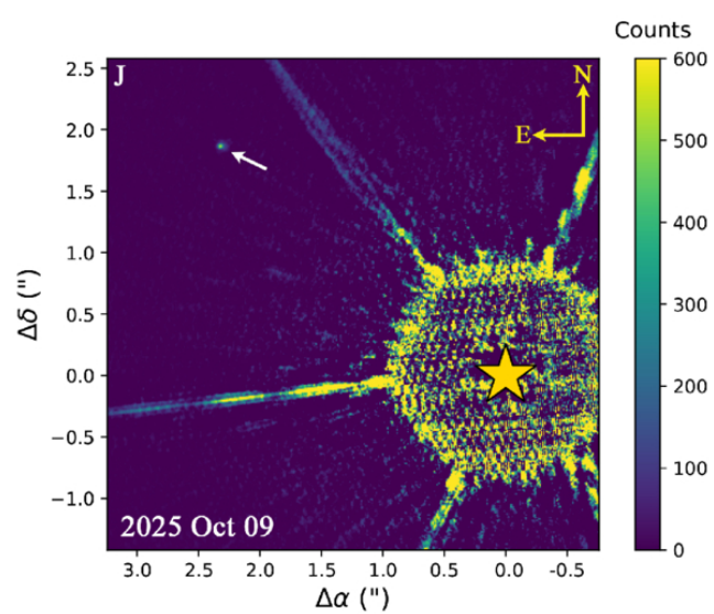
Epoch 4
