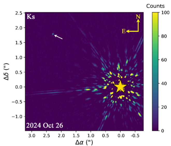
Epoch 3
