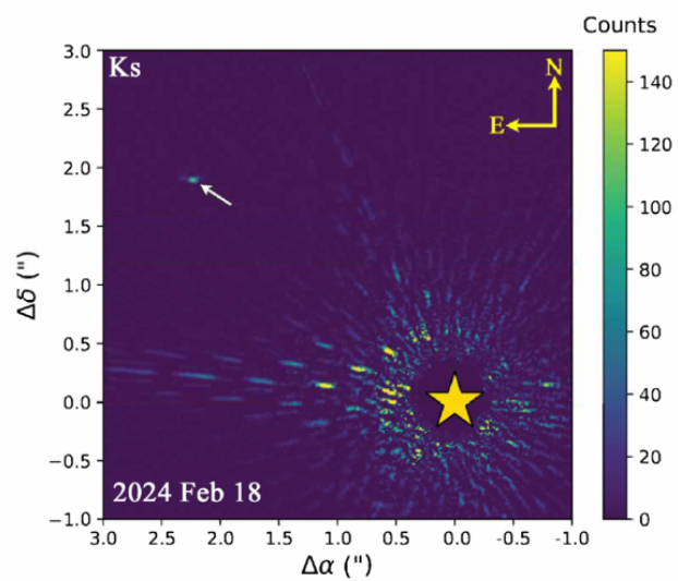
Epoch 2
