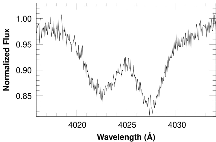
4026.358 Å He I
