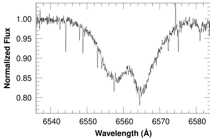
6562.79 Å H I
