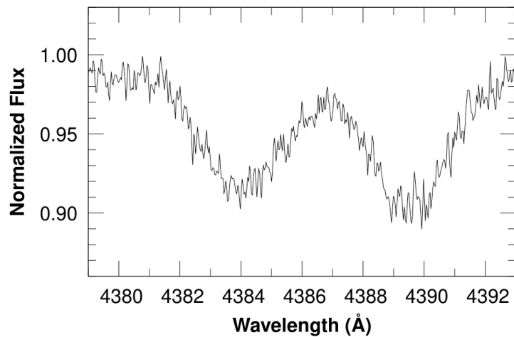
4387.929 Å He I
