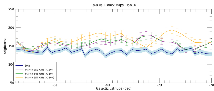
(c) Alice Row 16 Galactic Latitude
