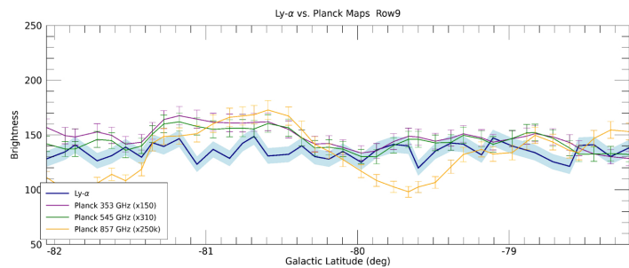
(a) Alice Row 9 Galactic Latitude
