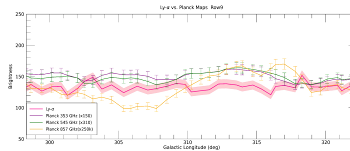
(b) Alice Row 9 Galactic Longitude
