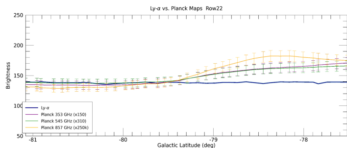
(e) Alice Row 22 Galactic Latitude
