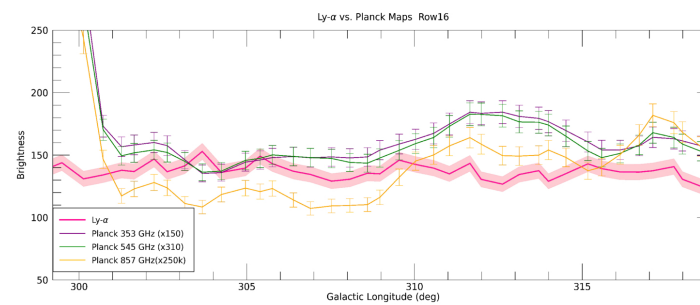
(d) Alice Row 16 Galactic Longitude
