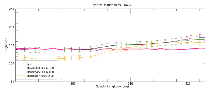
(f) Alice Row 22 Galactic Longitude
