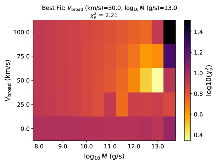
(d) Mg II only, T_{\text{iso}}=8,000 K
