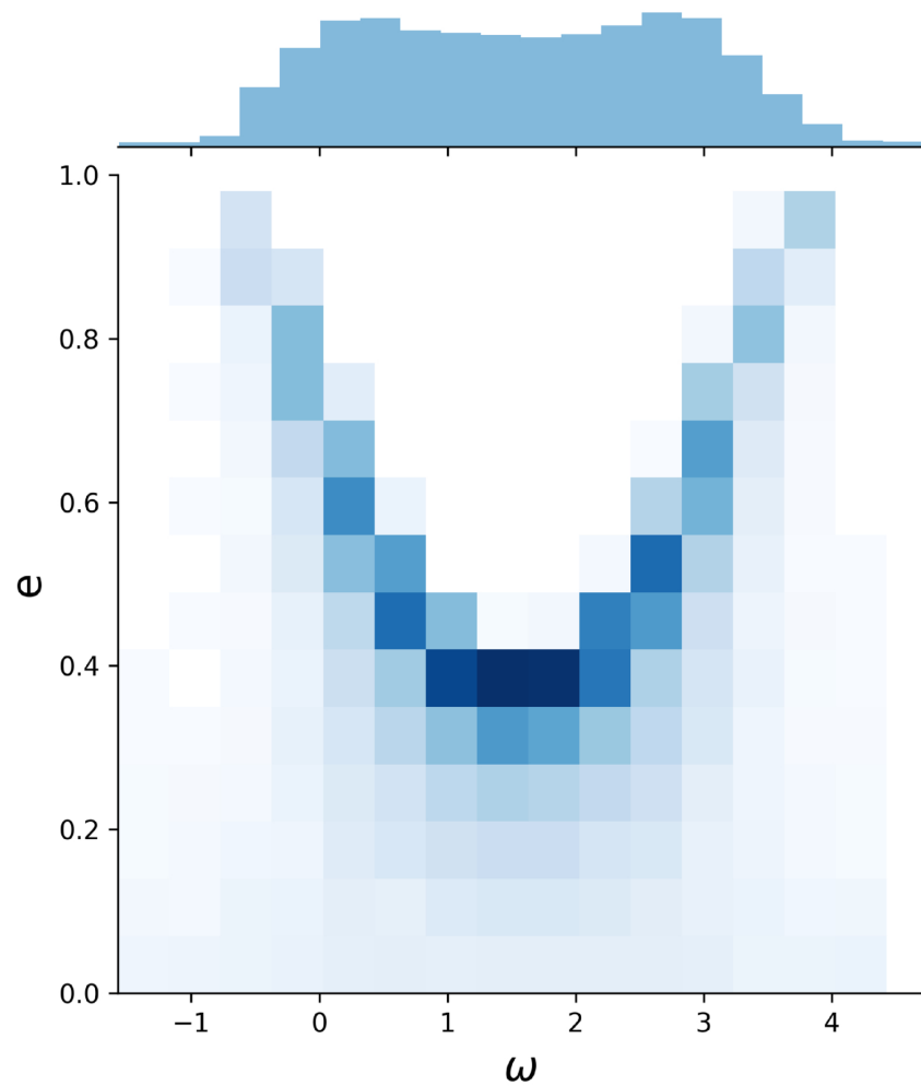
e - \omega posterior from Sagar et al. (2023)
