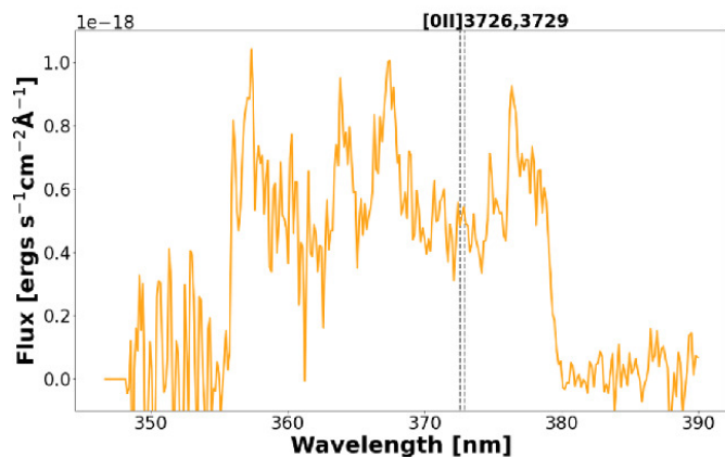
(d) SN1 sky emission
