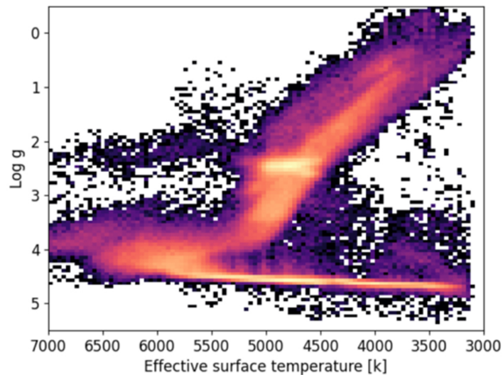
(b) Post uncertainty cut kiel diagram
