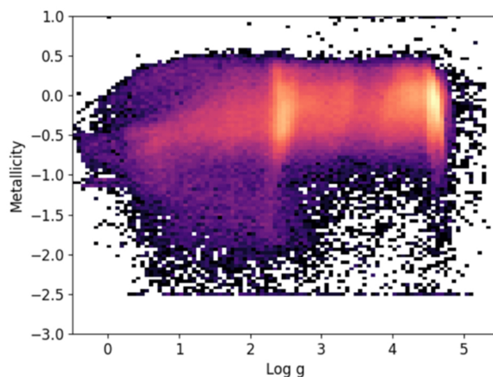
(d) Post uncertainty cut log g vs metallicity
