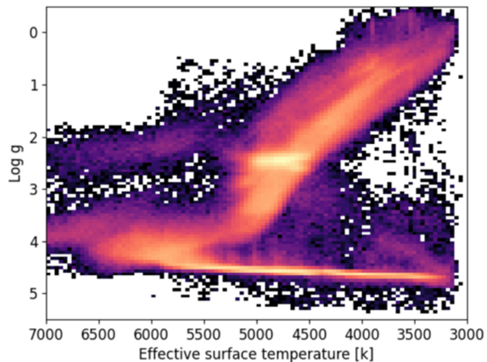
(a) Full data set kiel diagram
