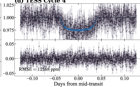
(d) TESS Cycle 4
