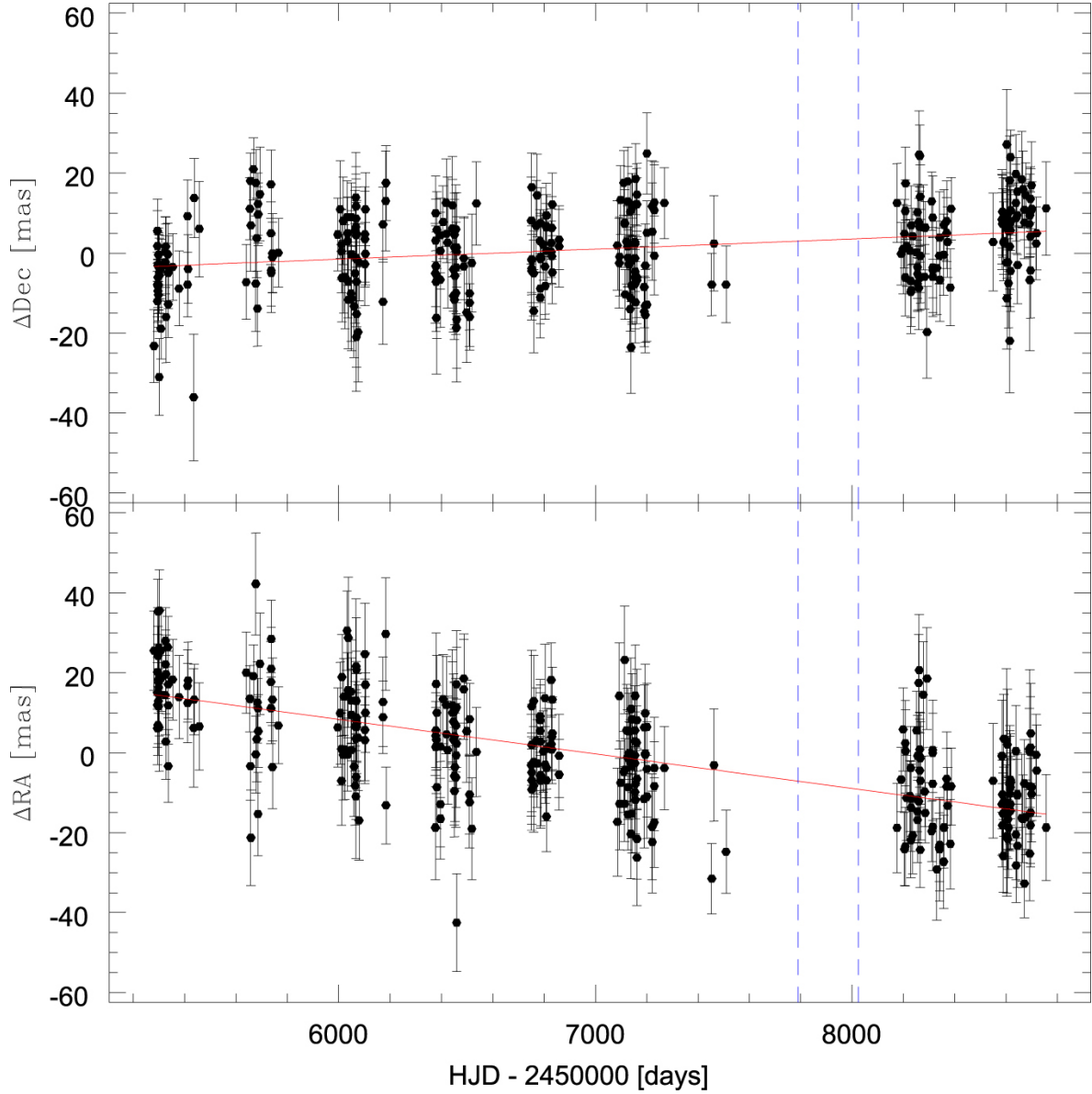
OGLE-2017-BLG-0406S
