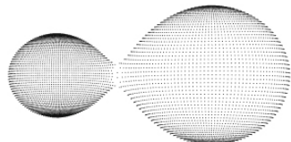
V646 Lac
