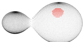
V539 Dra
