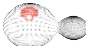
V816 Cep
