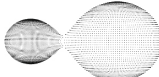
V596 Peg
