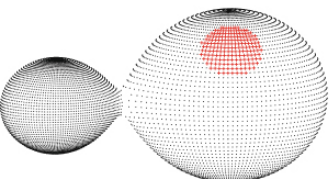
NSVS1768818
