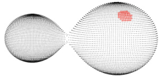
NSVS 3325547
