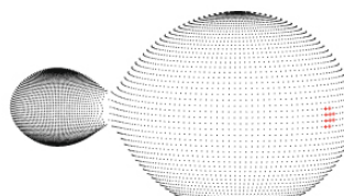
NSVS 3198272
