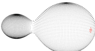
V619 Peg
