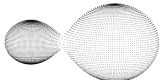
V1320 Cas
