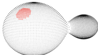
V1115 Cas
