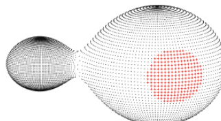
V509 Cep
