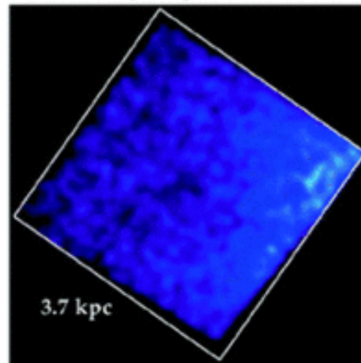
(d) Density Map of Red Stars
