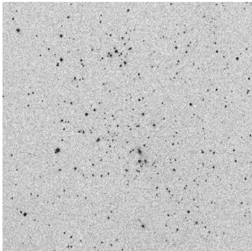
NSCJ122906+473720 zphot=0.3254 Ngals=66
