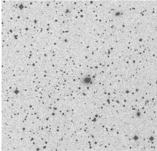
NSCJ172357+270033 zphot=0.1623 Ngals=90
