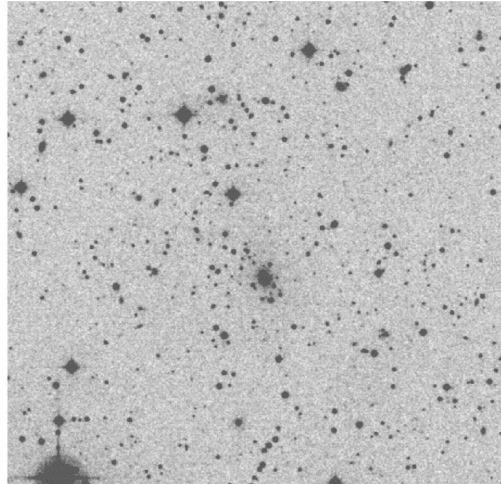
NSCJ172013+264028 zphot=0.2143 Ngals=69
