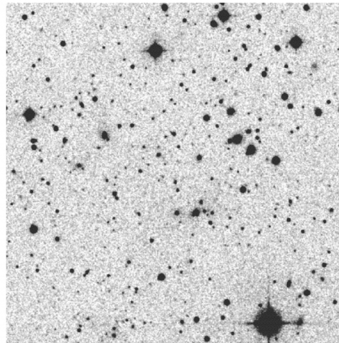
NSCJ081454+383306 zphot=0.1778 Ngals=67
