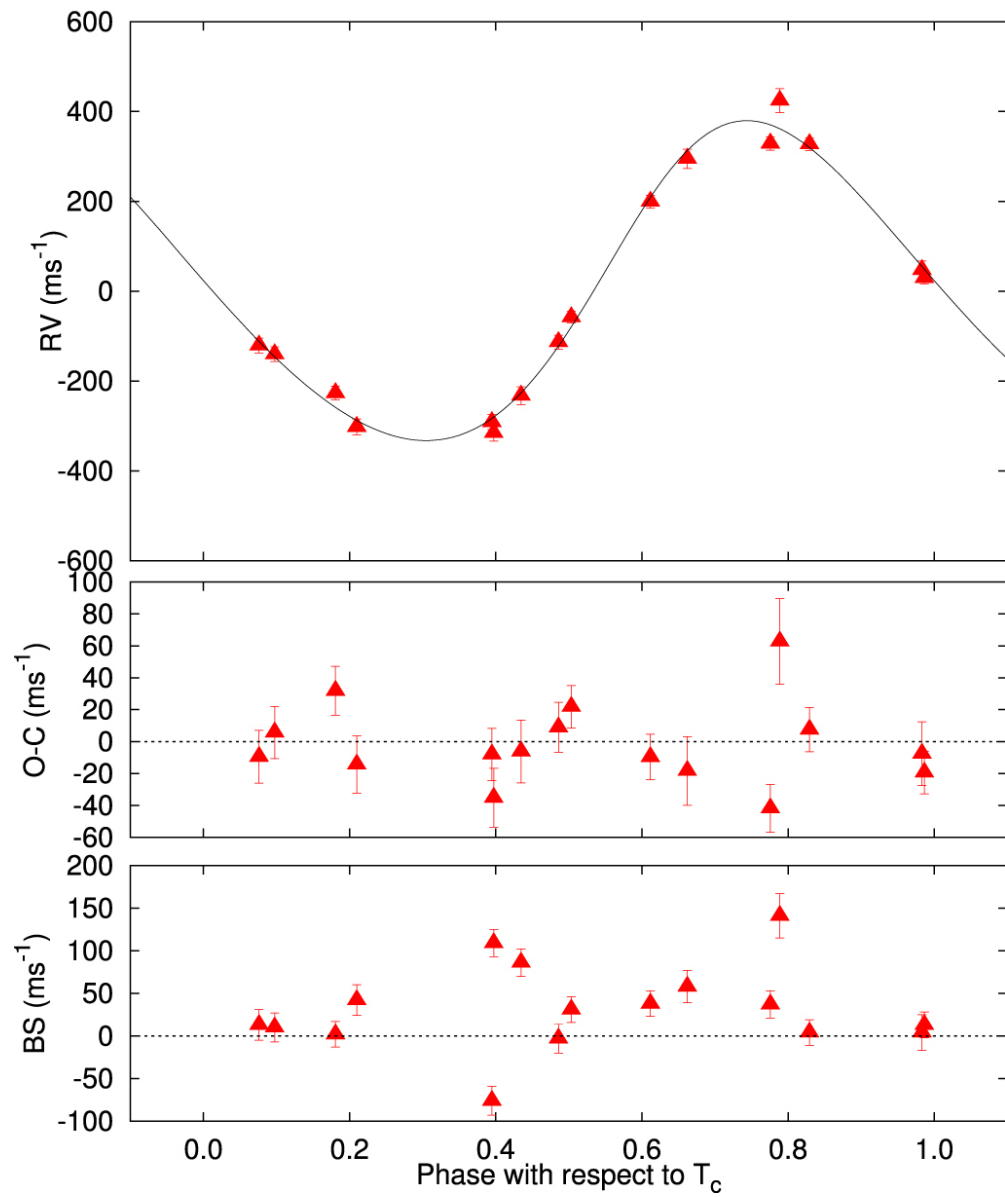
HATS-36
